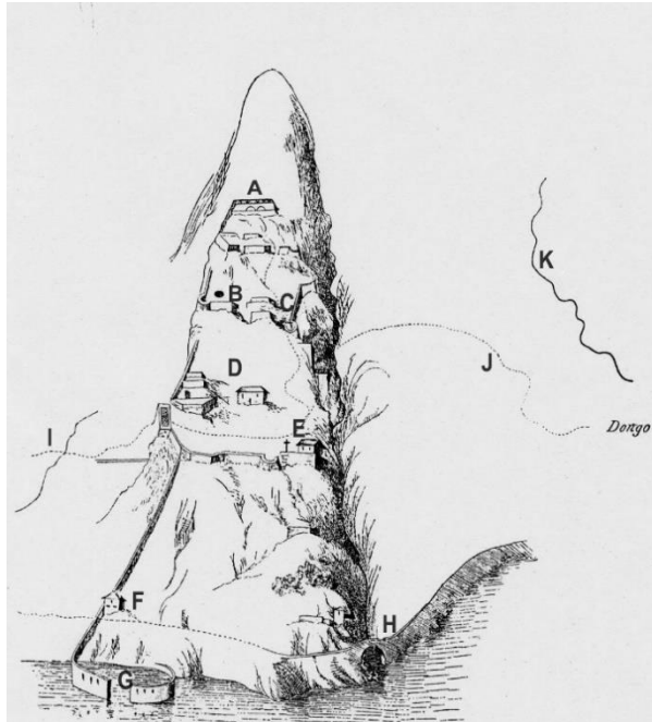
Fig. 4 Tekening van het kasteel van Musso. A) Uitgehakte geul die de slotgracht vormt, B) put, C) verblijven van de wacht, D) eerste niveau, E) kerk van S. Eufemia, F) wachtpost boven de haven, G) haven, H) brug met toegangspoort, I) weg naar Musso, J) weg naar D K) vallei van Dongo met de weg naar Bellinzona
